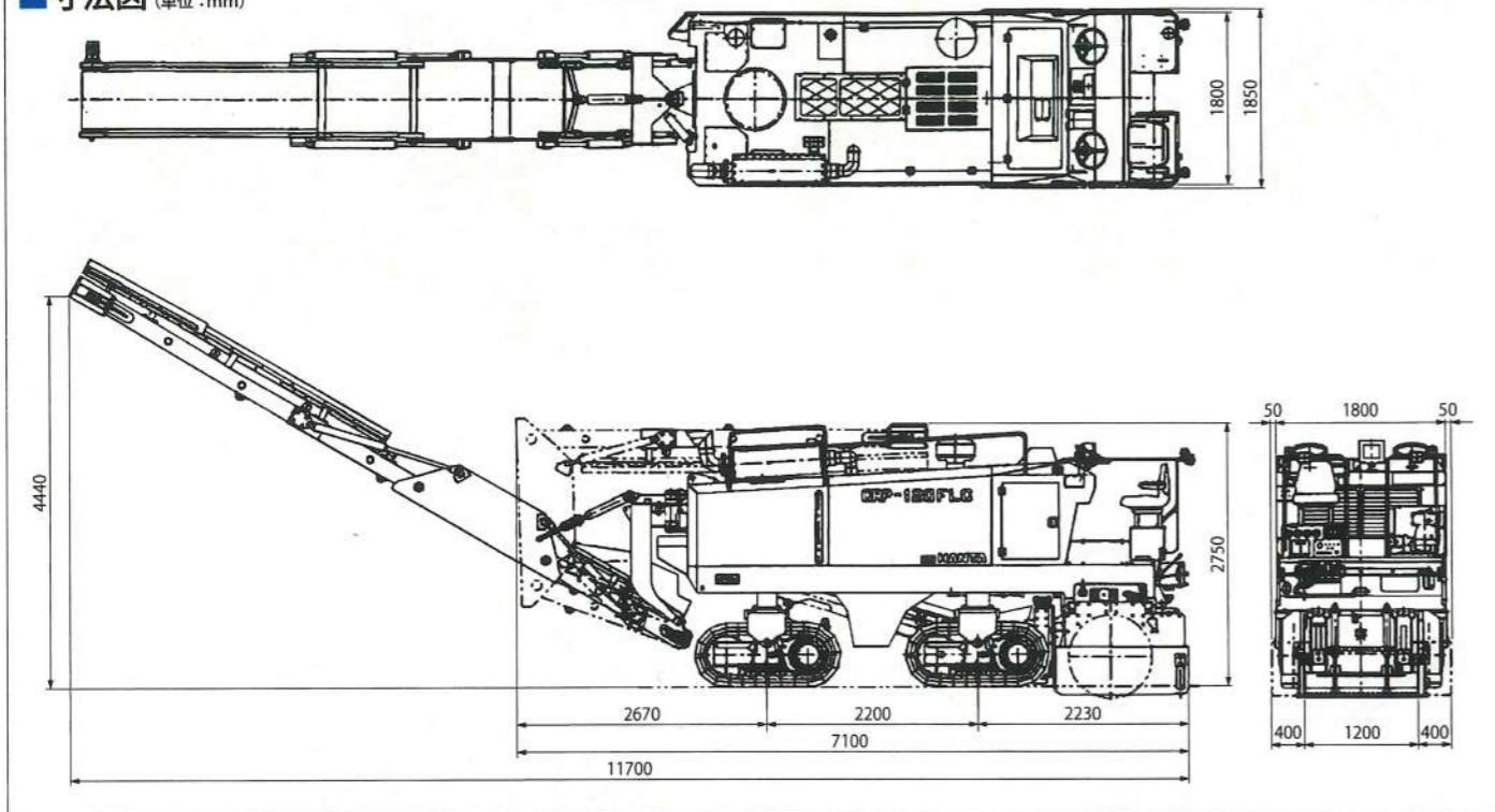
■CRP-120FLC主要諸元表
